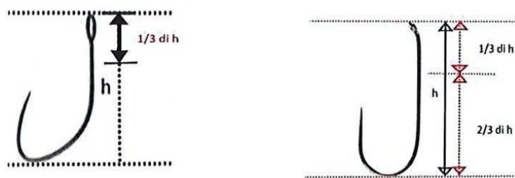
2. ábra: A horog súlyozását – az ábrán bemutatott módon – a horogszár felső 1/3-ában lehet elhelyezni.
